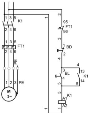
ESQUEMA DE LIGAÇÃO
