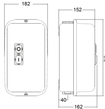
DIMENSÃO QCX2-40/QCX2-50/QCX2-65/QCX2-80 e QCX2-95
