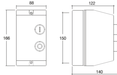
DIMENSÃO QCX2-09/QCX2-12 e QCX2-18
