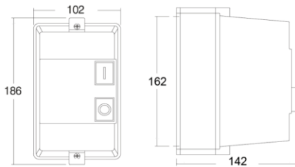
DIMENSÃO QCX2-25 e QCX2-32
